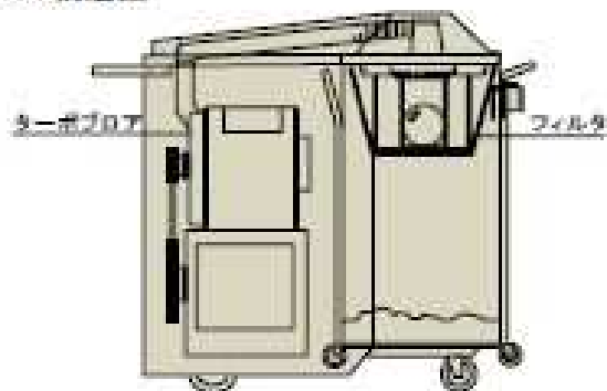
NWV構造図
