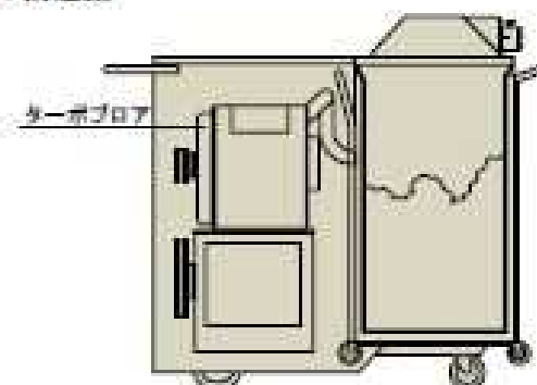
NTV構造図
